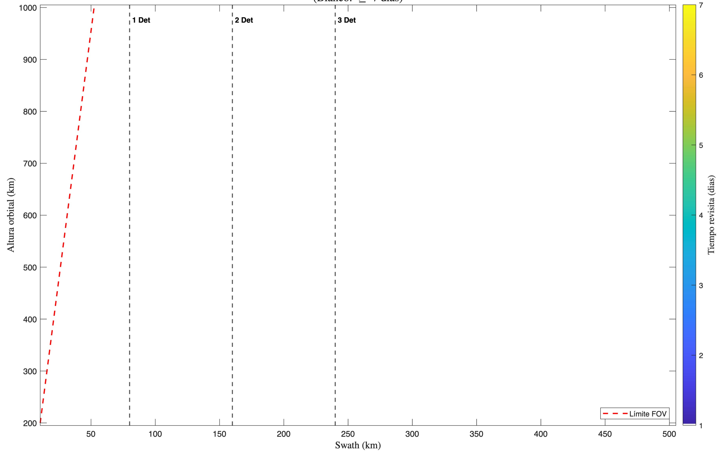
Tiempo Revisita - 3 Satellite(s); 1 Telescopio(s): Cassegrain; Detector 3 (Blanco: \geq 7 días)
